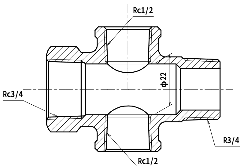
A-A断面図
